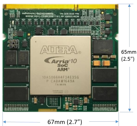
Fig. 3 SOC MPEG Codec Module
